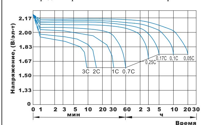
Рис 3. Разрядные кривые постоянным током при 25°C
