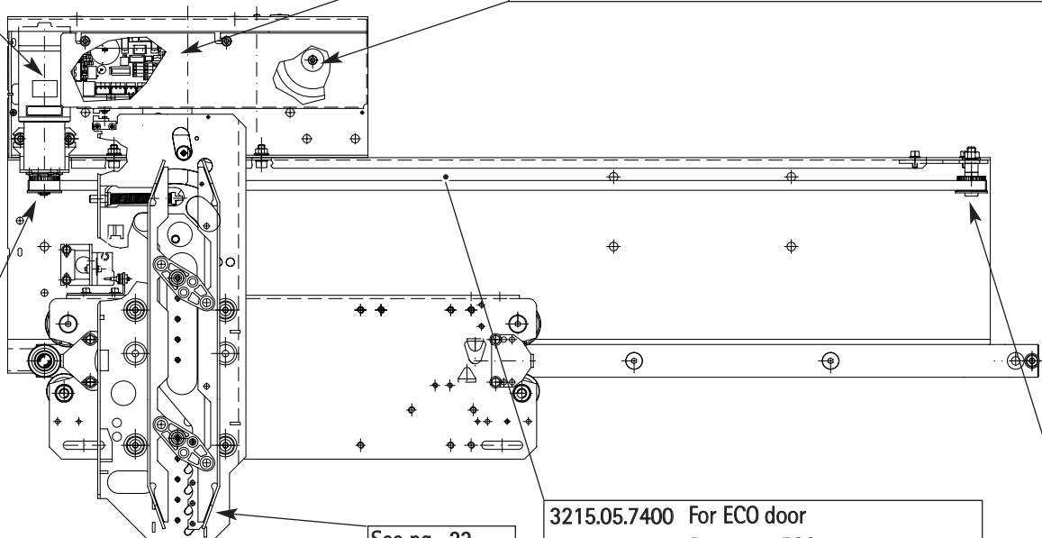
3215.05.0041 Motor pulley for ECO Puleggia motore per ECO
