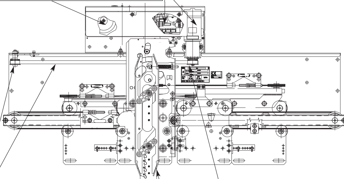
3215.05.7400 For ECO door Per porta ECO
