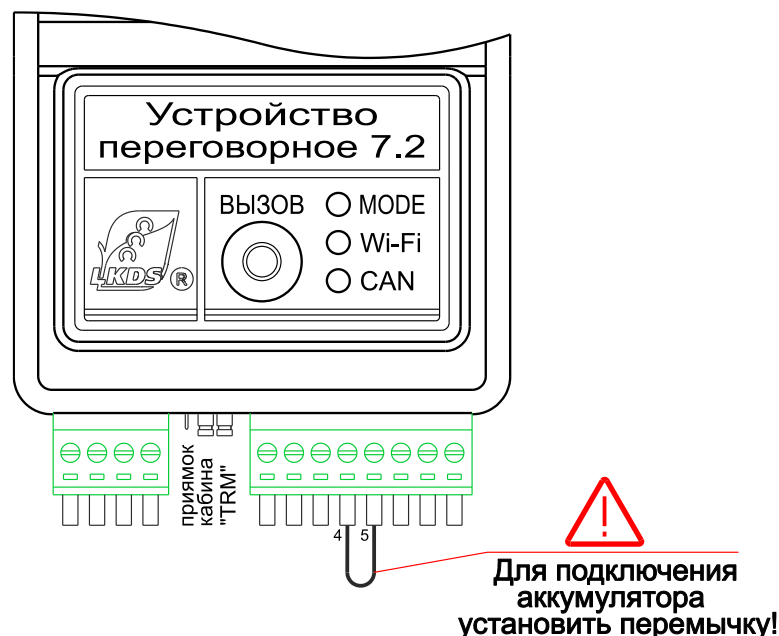
Рисунок 12. Подключение аккумуляторной батареи переговорного устройства и установка джамперов «Кабина/Приемок»
