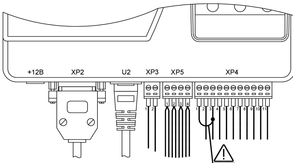
Рисунок 11. Подключение аккумуляторной батареи лифтового блока
